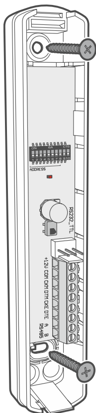
Obr. 6. Montáž zadní části krytu.
