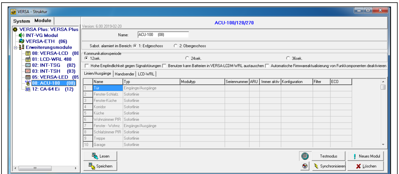
Abb. 25. Programm DLOADX: Einstellungen des Funkbasismoduls im System VERSA.
