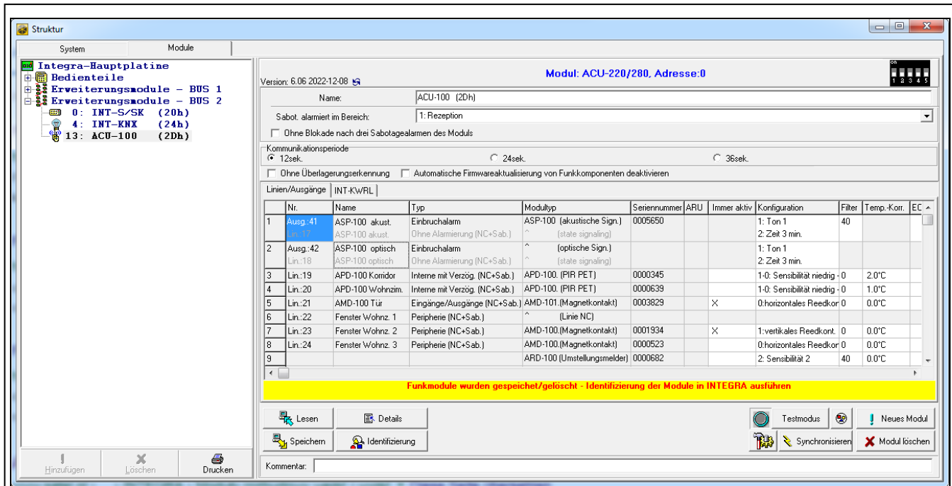
Abb. 23. Programm DLOADX: Informationen, die nach der Registrierung eines neuen Moduls im Funkbasismodul im System INTEGRA angezeigt werden.
