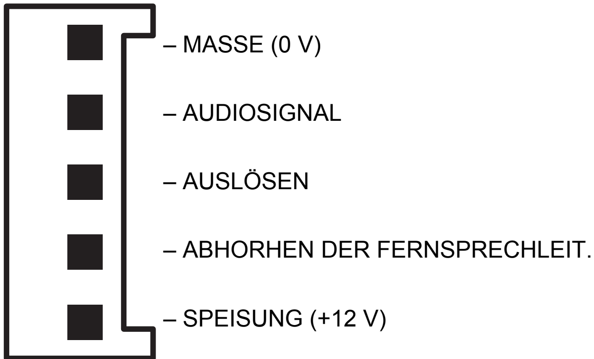
Abb. 1. Einteilung von Signalen an Klemmen des SM-2 Moduls.
