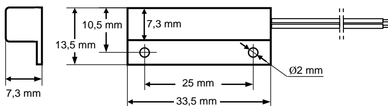
Fig. 1 Interruptor del contacto "reed" del contacto K-1 2E en la caja de plástico.
