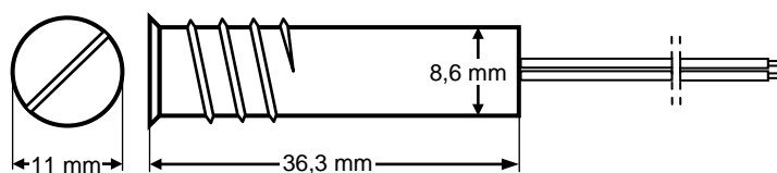
Fig. 3 Interruptor del contacto "reed" del contacto K-3 2E en la caja de metal.
