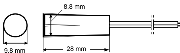
Fig. 1 Interruptor del contacto "reed" del contacto K-1 2E en la caja de plástico.
