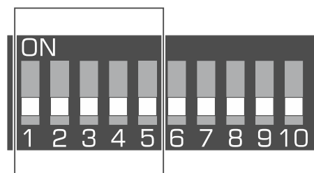
Fig. 3. Interrupteurs pour définir l'adresse du contrôleur dans le système INTEGRA.
