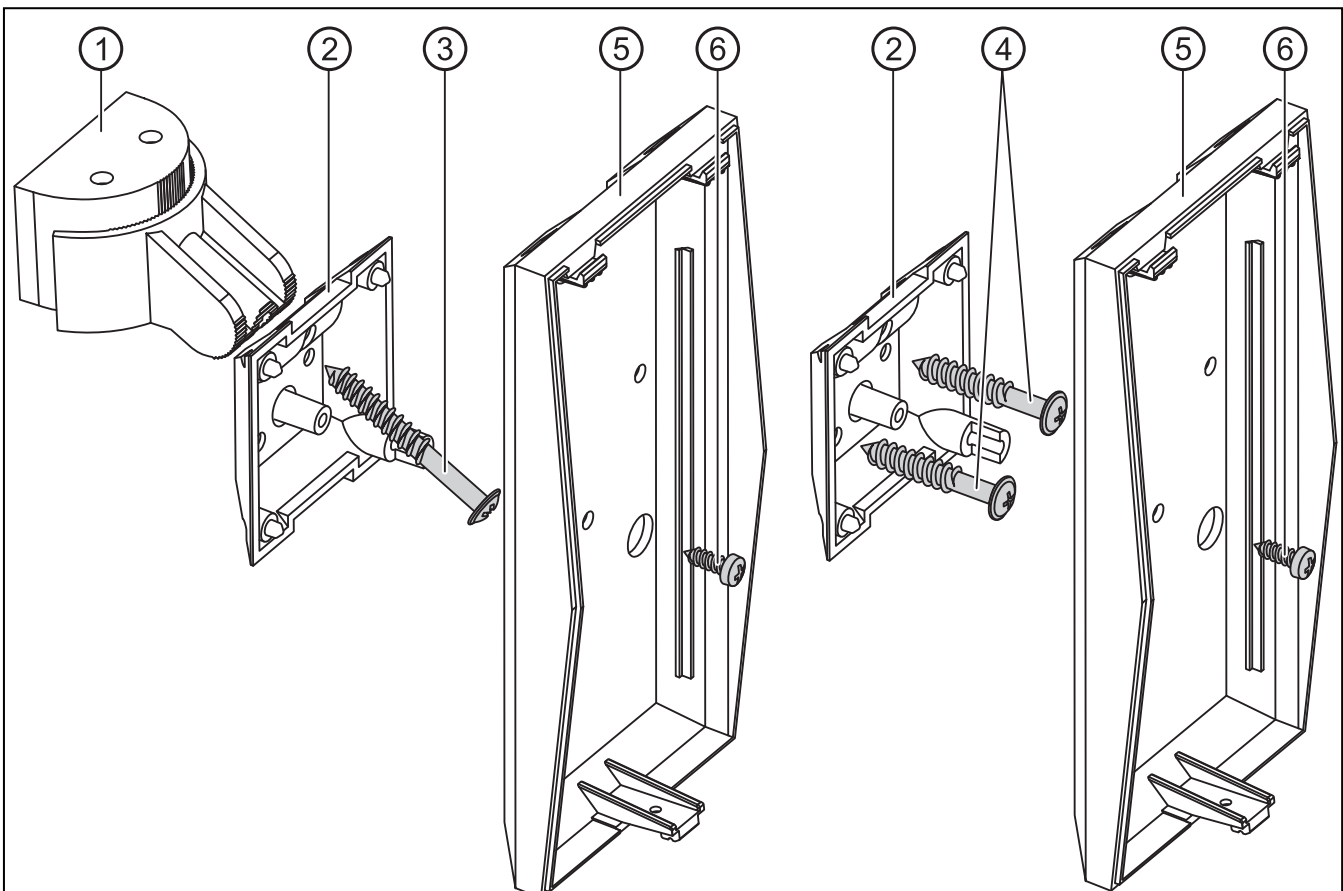
2. Ábra. Az érzékelő szerelése tartóra vagy közvetlenül a falra. 1 – tartó. 2 – hátsó tamper egység. 3 – a hátsó tamper egység tartóhoz rögzítő csavarja. 4 – a hátsó tamper egység falhoz rögzítő csavarjai. 5 – az érzékelő ház hátsó része. 6 – az érzékelő ház hátsó részét a hátsó tamper egységhez rögzítő csavar.
