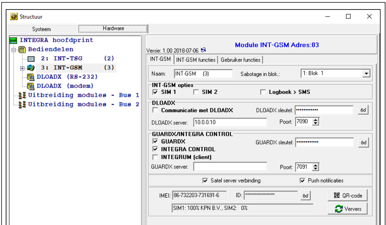
Afb. 9. DLOADX programma: instellingen van de INT-GSM LTE module welke direct aangesloten is op het INTEGRA / INTEGRA Plus alarmsysteem.
