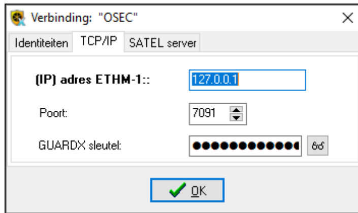
Afb. 22. GUARDX programma: "TCP/IP" tabblad in het "Verbinding" scherm.
