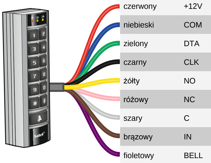
Rys. 2. Przewody klawiatury.
