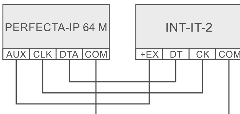
Rys. 10. Podłączenie modułu INT-IT-2 do centrali.
