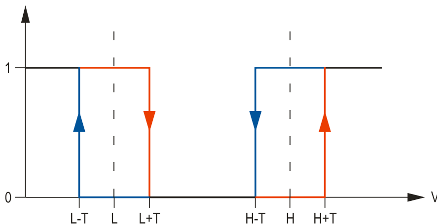
Рис. 10. Способ работы аналогового входа. 0 – отсутствие нарушения. 1 – нарушение.
