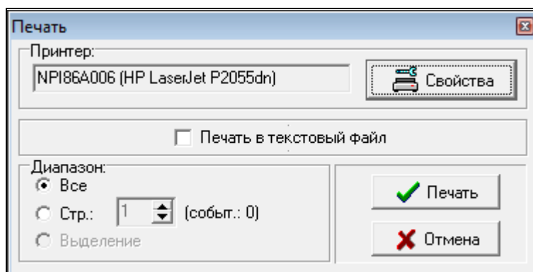
Рис. 20. Окно «Печать».
