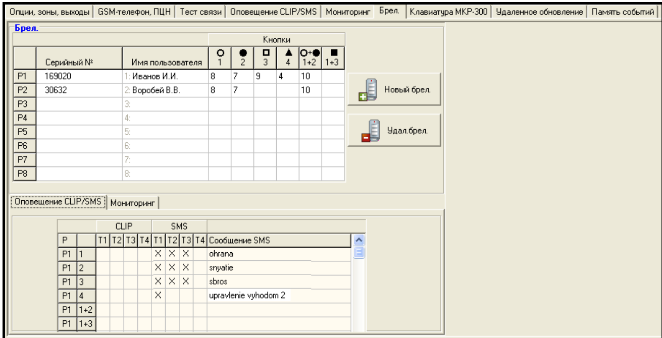
Рис. 15. Вкладка «Брелоки».
