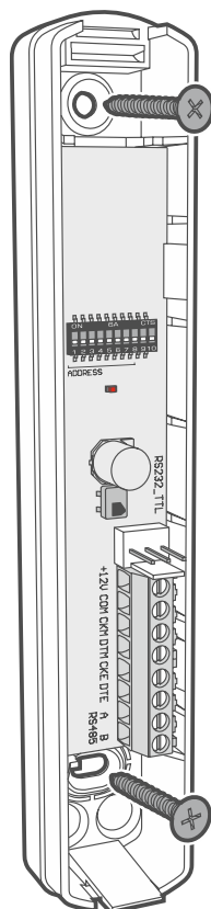
Рис. 6. Установка основания корпуса.
