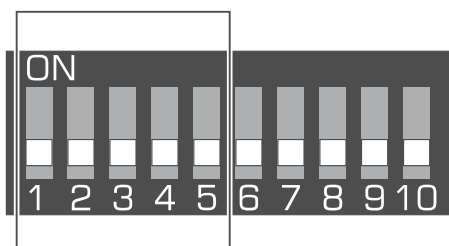
Рис. 3. Переключатели, предназначенные для установки адреса, если контроллер подключен к прибору INTEGRA / INTEGRA Plus.
