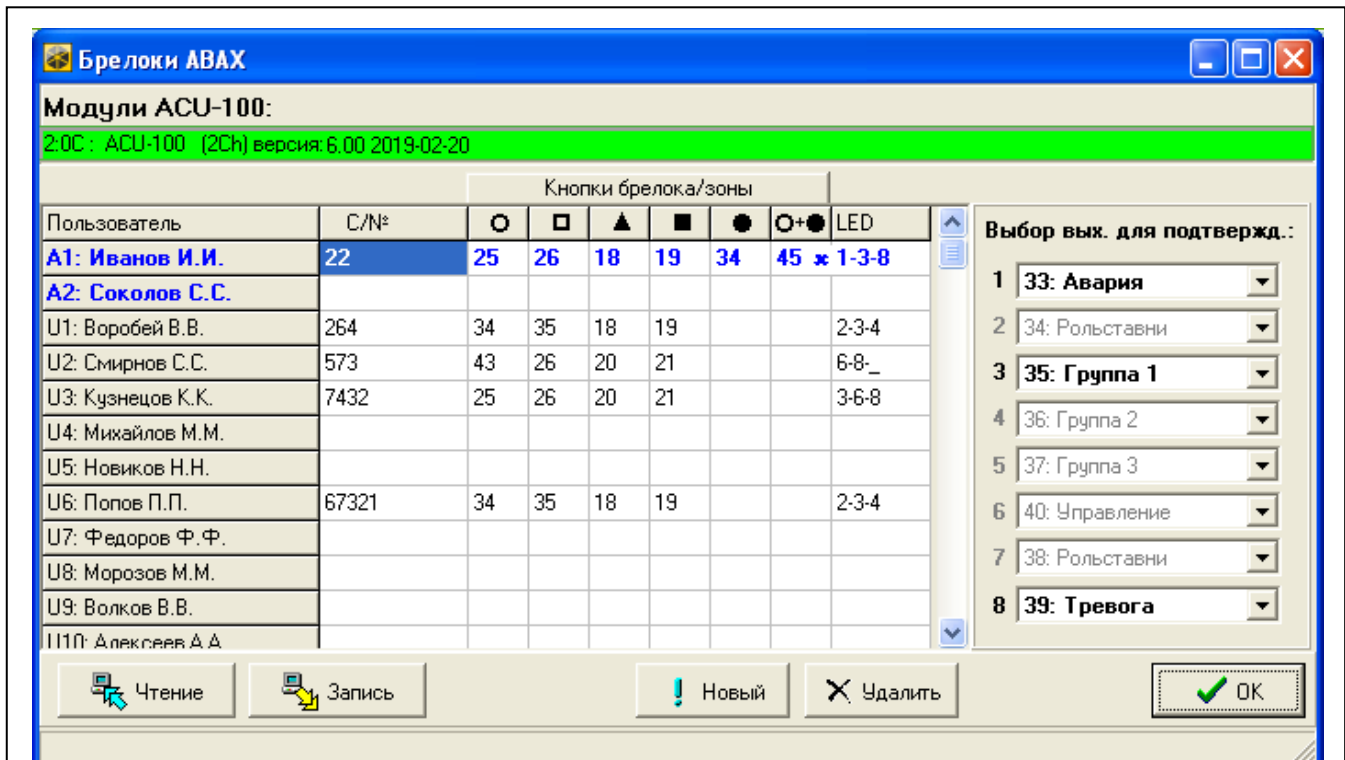
Рис. 26. ПО DLOADX: управление брелоками, если контроллер подключен к прибору INTEGRA / INTEGRA Plus.
