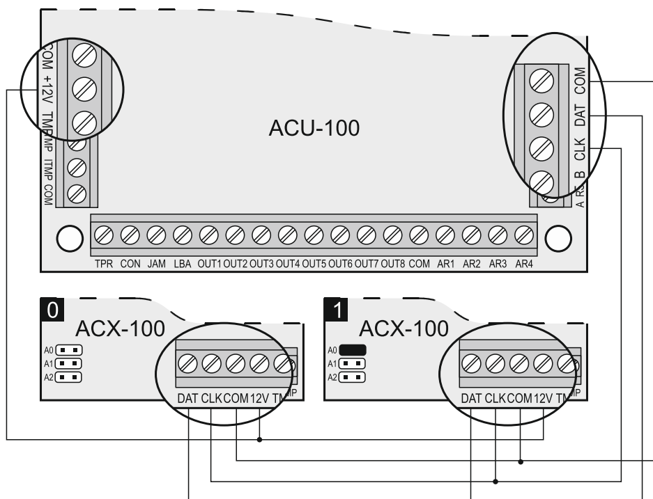
Рис. 6. Пример подключения 2 модулей ACX-100 (адреса: 0 и 1) к контроллеру ACU-100.
