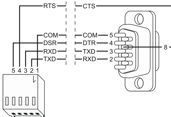
Рис. 5. Подключение ПК к последовательному порту ACU-100. С левой стороны вид разъема PIN5. С правой – разъем типа «мама» DB-9 со стороны точек пайки.
