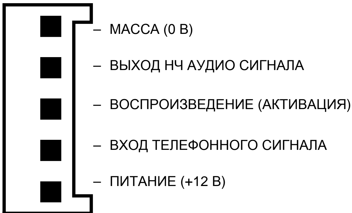
Рис. 1. Разводка контактов разъема модуля голосового оповещения SM-2.
