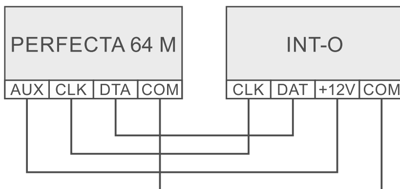
Obr. 10. Pripojenie expandéra INT-O na ústredňu.
