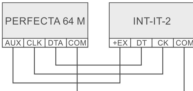
Obr. 11. Pripojenie modulu INT-IT-2 na ústredňu.
